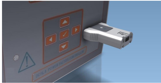
Adaptador de programación USB ref. CX01. Adaptador de programación WiFi ref. CX02. USB programming dongle code CX01. WiFi programming dongle code CX02
