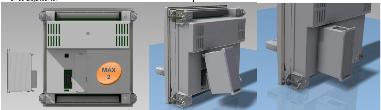
Montaje de los módulos de expansión
